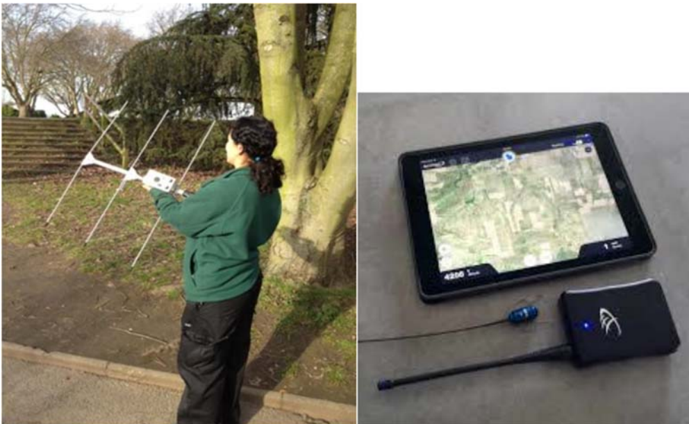
Figuras 17 y 18 muestran un receptor común que se usa para localizar un transmisor y un nuevo sistema de GPS que se vincula con la tecnología de GPS de smartphones y tablets.
